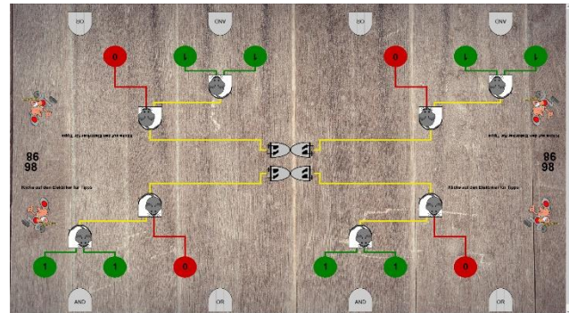
Abbildung 2: kooperatives Multitouch-Lernspiel
